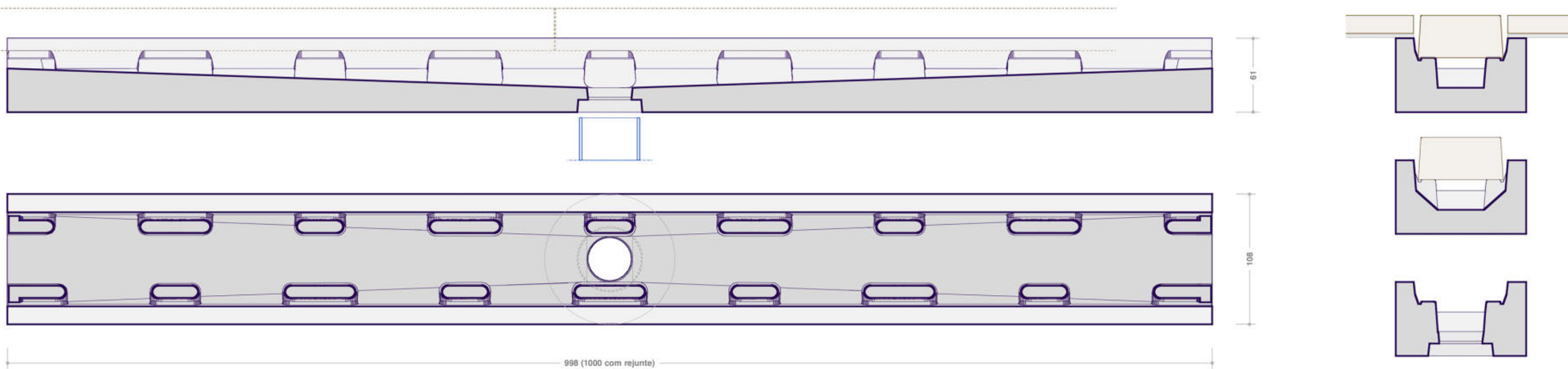
Peça Canaleta em Concreto (998x108x61)
